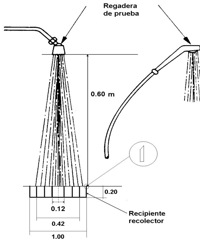
Figura 3. Eficiencia de la regadera
