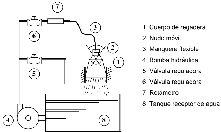
Figura 5. Instalación de prueba
